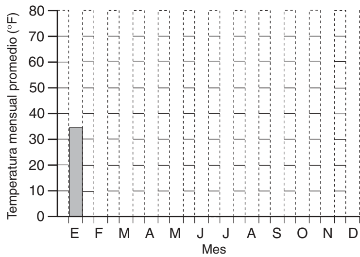
Temperaturas mensuales promedio de la zona climatológica 5
