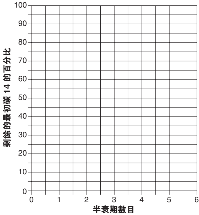
碳 14 的放射性衰變
